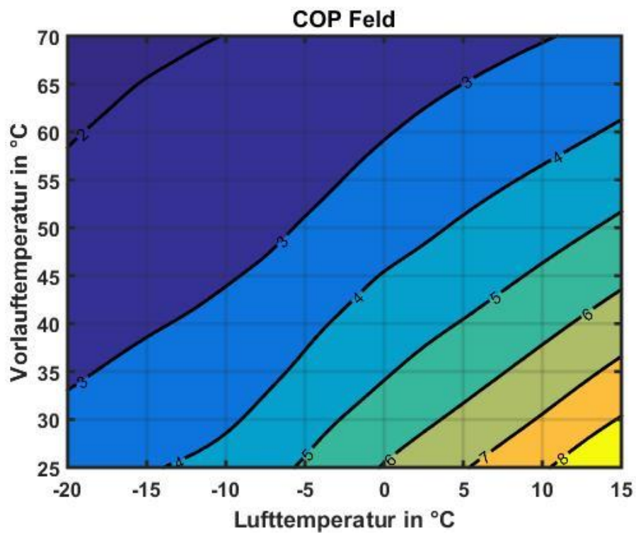
Abbildung 11: EU13L bei 9kW Heizleistung
