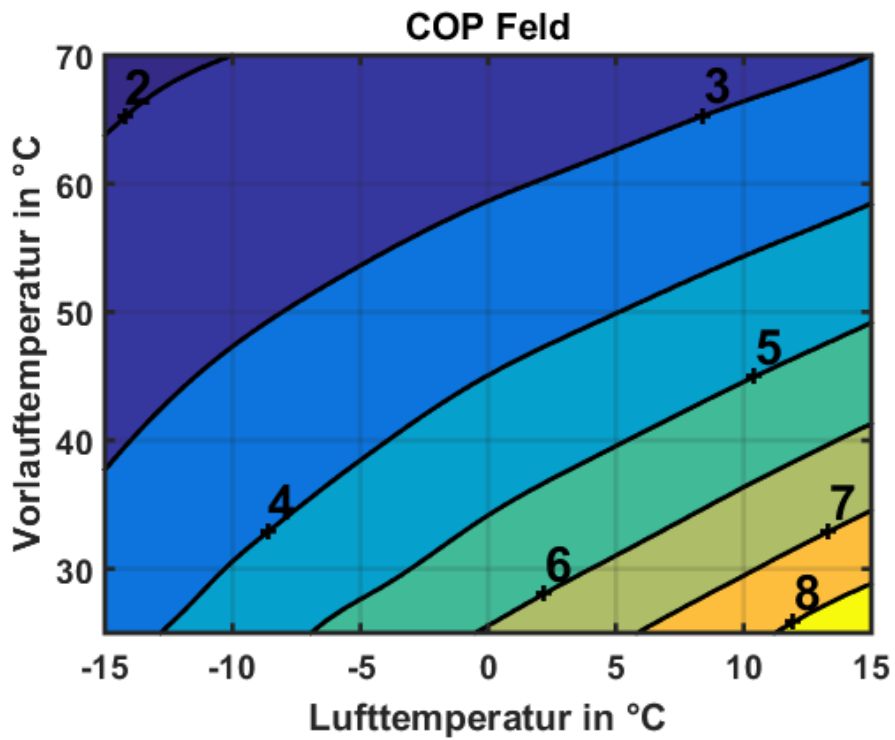
Abbildung 10: EU15L bei 11kW Heizleistung
