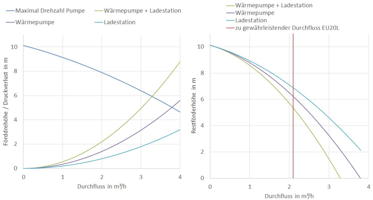
Abbildung 14: Pumpenkennlinie, Anlagenkennlinie und Restförderhöhe EU20L
