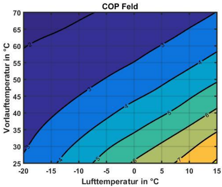
Abbildung 12: EU08L bei 6kW Heizleistung
