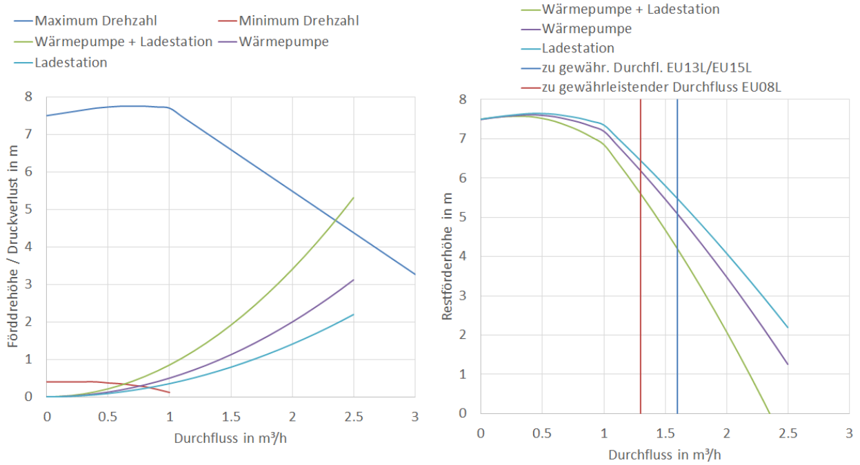
Abbildung 13: Pumpenkennlinie, Anlagenkennlinie und Restförderhöhe EU20L
