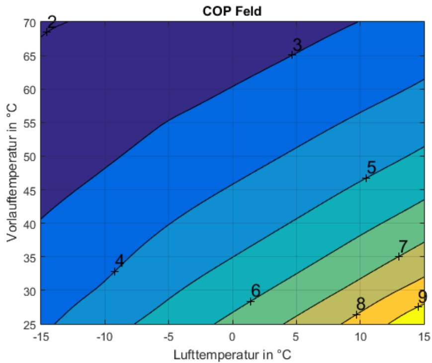
Abbildung 9: EU20L bei 14kW Heizleistung
